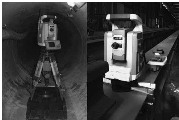
Spezielle Tachymetermontagen beim Kanal- und Gleisbau.
