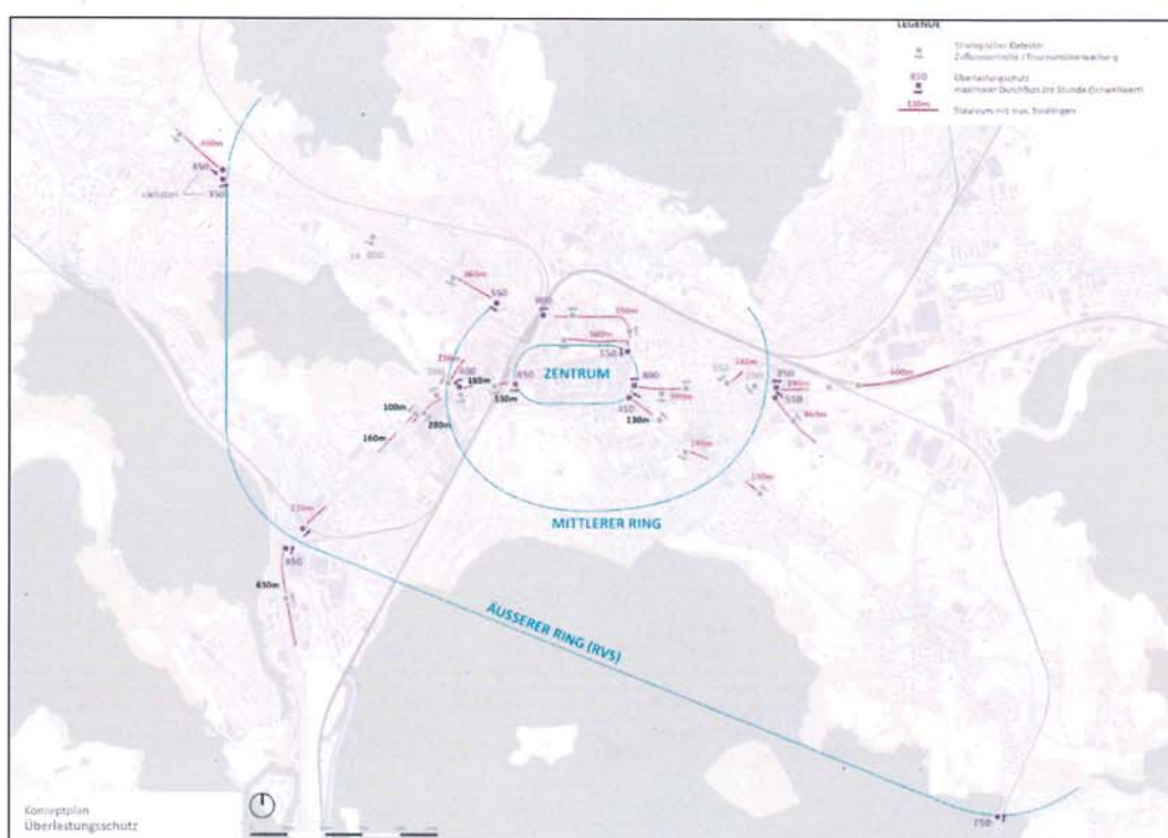
Abbildung 7: Konzept Überlastungsschutz
