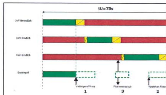
Abbildung 5: Schema der Buspriorisierung am Einzelknoten mittels Verlängern der Grünphase (1), Phaseneinschub (2) oder Vorziehen der Grünphase (3)
