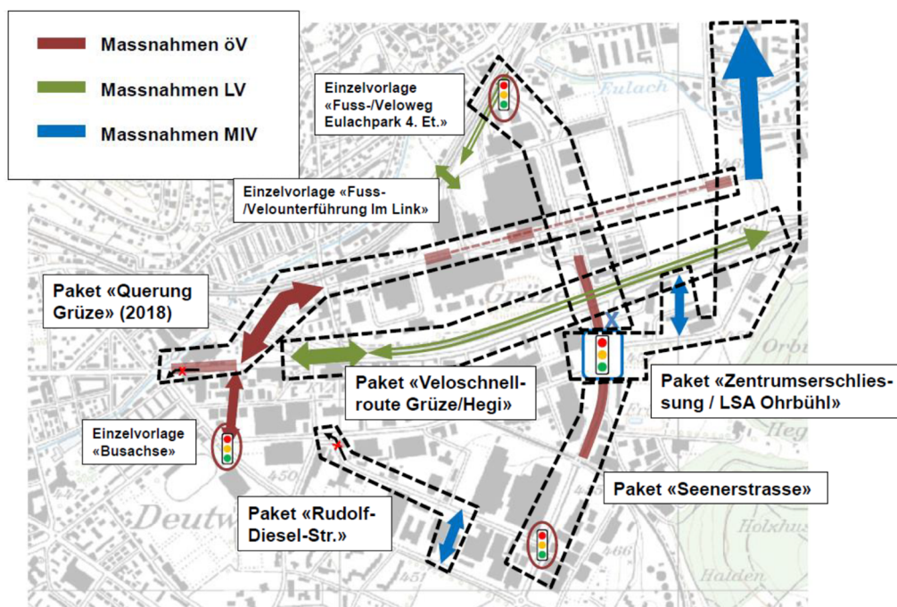
Abbildung: Paketbildung für die Verkehrsprojekte im Raum Neuhegi-Grüze
