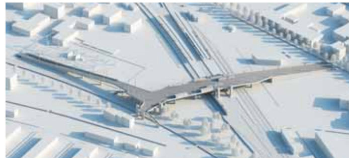
Querung Grütze ohne möglicher Bebauung
