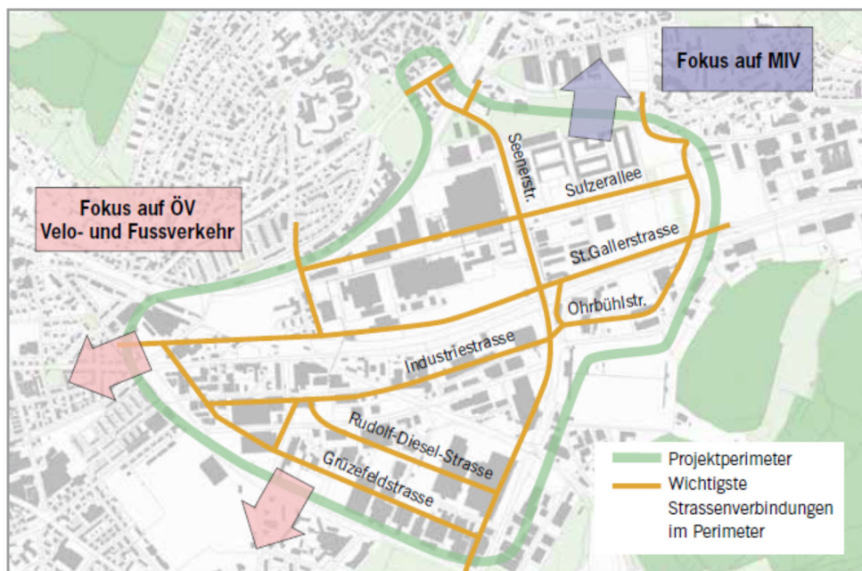
Abbildung: Grundprinzip des Gesamtverkehrskonzepts Neuhegi-Grüze
