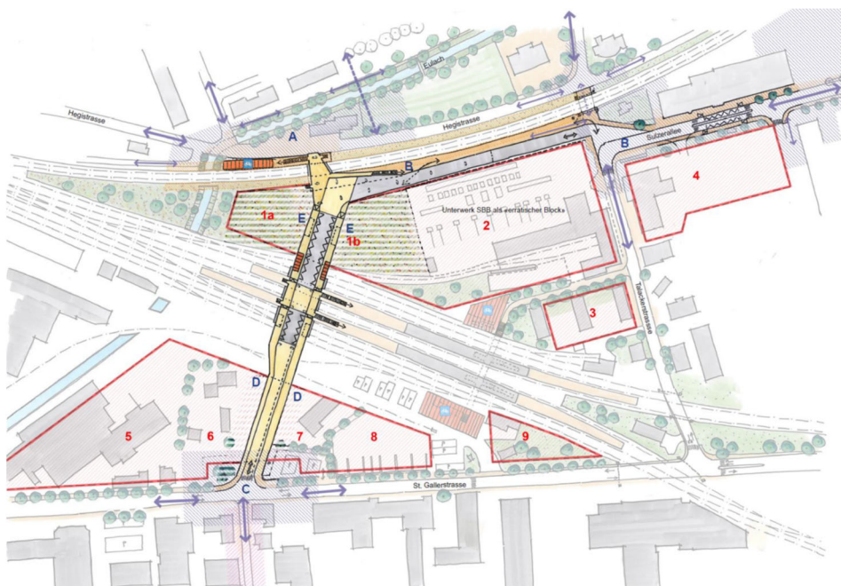
Abbildung: Situationsplan
