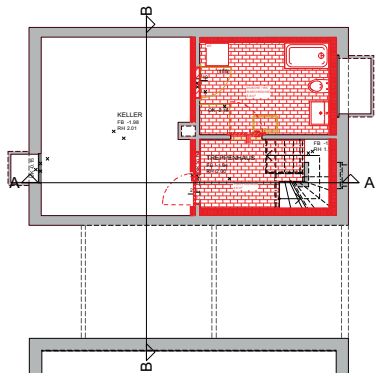
Grundriss UG / OG 1:200
