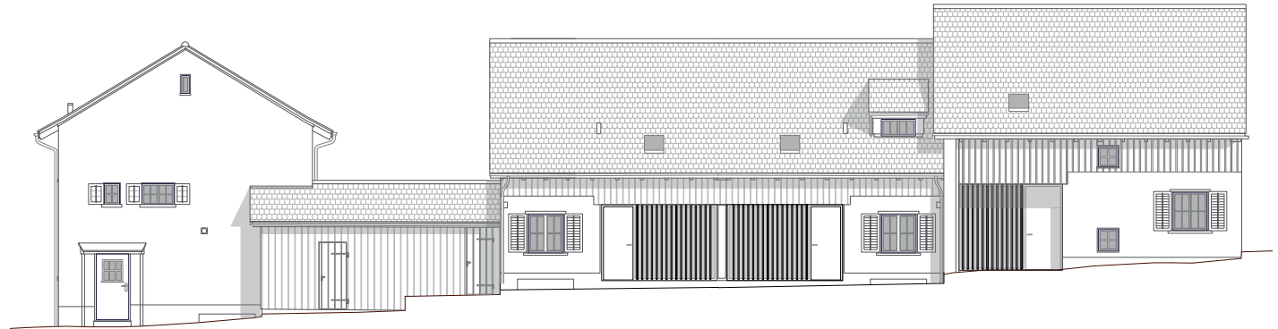
Häuserzeile N10 / Typ G,E,E,J Nordfassade
