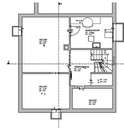
Typ L (Bestand 3 Nasszellen)
